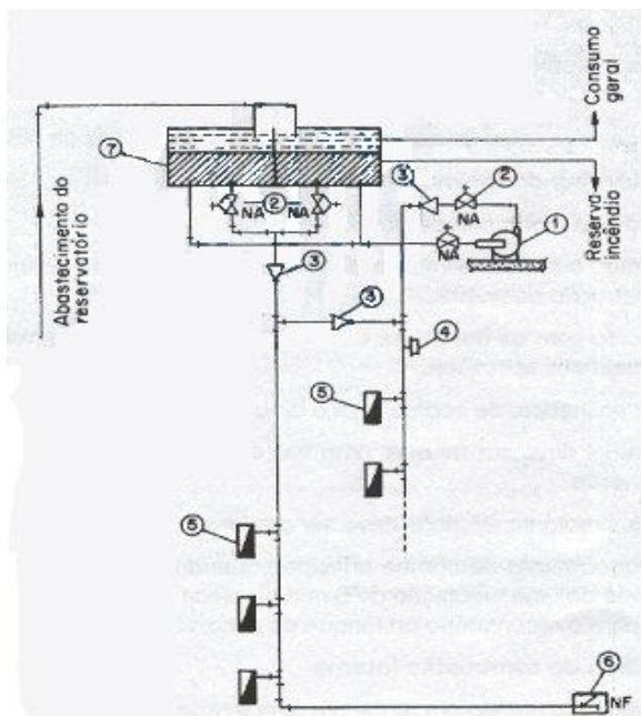
Figura apoio a C.6 - Esquema de instalação de bomba de reforço abastecendo os pontos de hidrantes ou mangotinhos mais desfavoráveis considerados no cálculo, (prumada específica)
