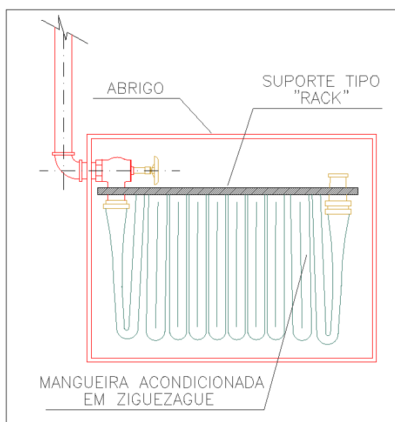
Figura 3 - Suporte para mangueira tipo "rack"
