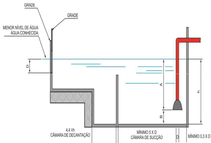
Figura B.5 – Alimentação natural de reservatório por canal
