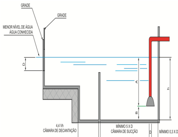
Figura B.4 - Alimentação natural do reservatório de incêndio
