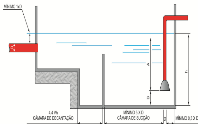
Figura B.6 – Alimentação natural de reservatório por conduto
