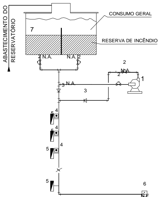
Figura apoio a C.5 - Esquema de instalação de bomba de reforço abastecendo os pontos de hidrantes ou mangotinhos mais desfavoráveis considerados no cálculo, por uma só prumada
