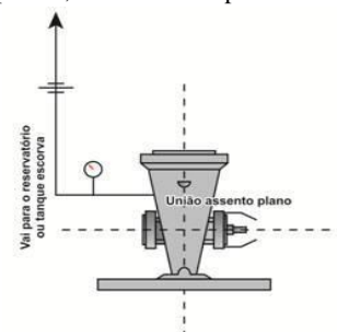
Figura C.7 – Arrefecimento da bomba principal elétrica.
