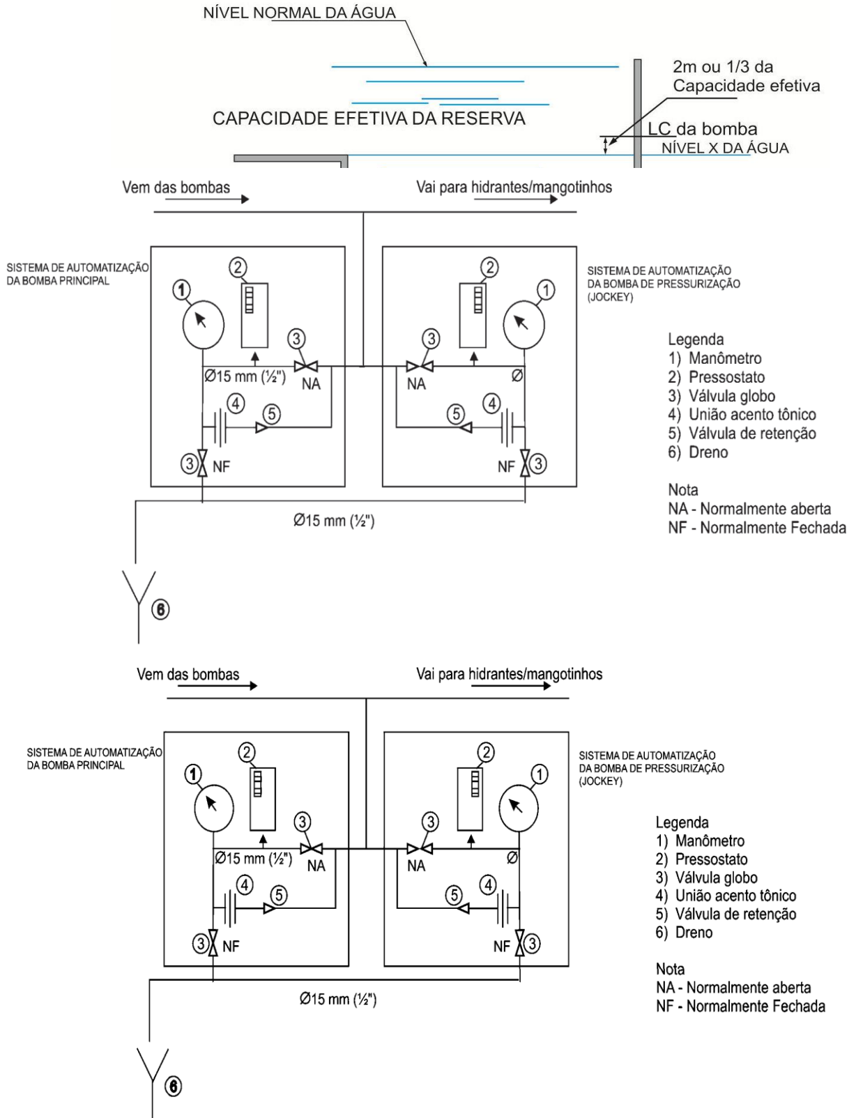
Figura C.2 – Cavalete de automação das bombas principal e de pressurização
