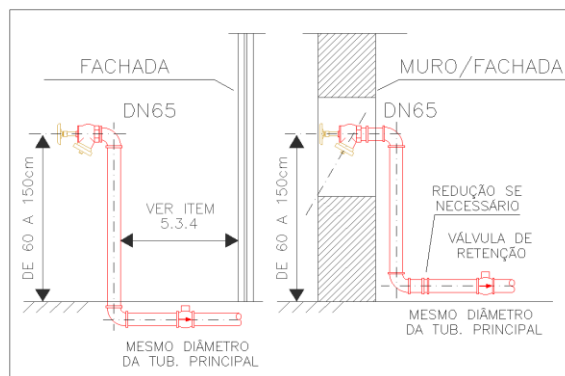
Figura 1 - Dispositivo de recalque, para o CBMRR, do Tipo coluna.
